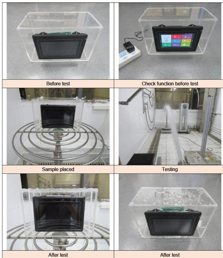
图 6-5 防水测试图
