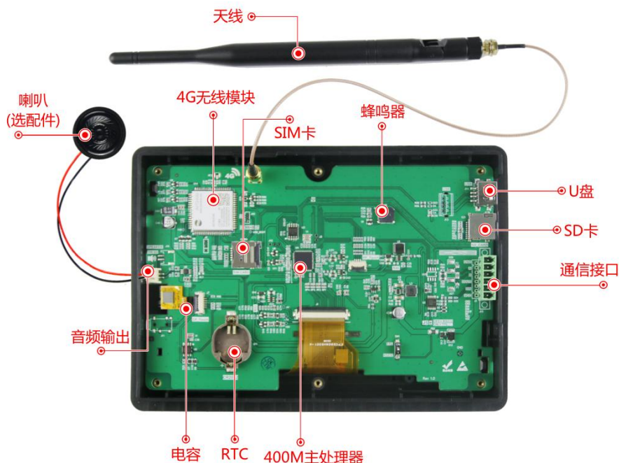
图 1-2 硬件配置图
